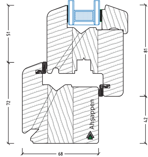
68 mm 45 BİRLEŞİM ULTAES SERİSİ
